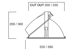
(d) DW Series: TC-DEL CFL Wallwasher
